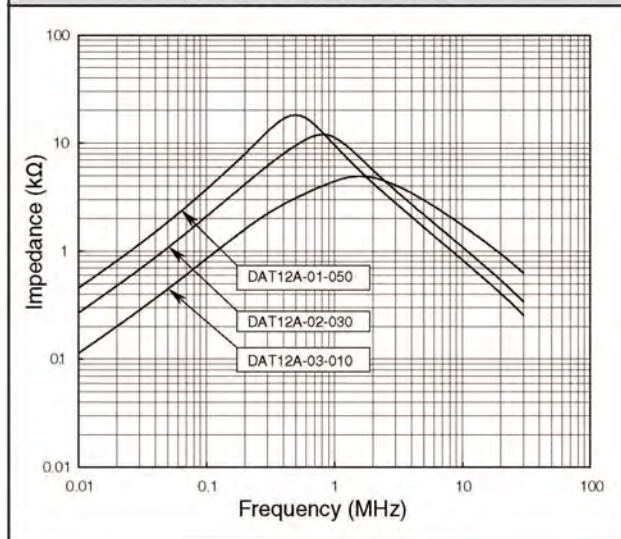
阻抗特性 (代表例)
